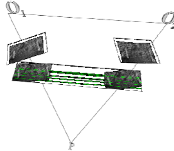
Fig. 3. : Epipolar rectification
